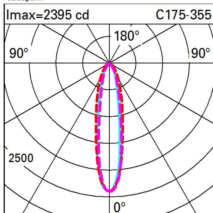
Polardiagramm
